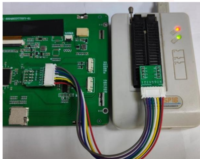
图 11.5 存储芯片与烧录器连接图
